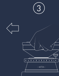
3. Aufsetzen des Einfülltrichters durch Drehen
